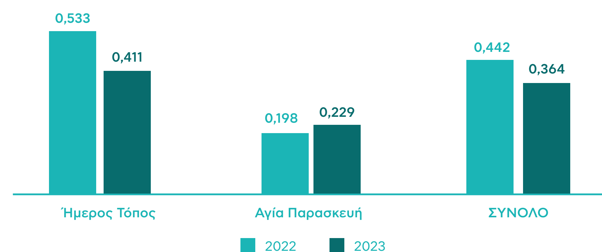
ΕΝΤΑΣΗ ΚΑΤΑΝΑΛΩΣΗΣ ΝΕΡΟΥ ΑΝΑ ΕΓΚΑΤΑΣΤΑΣΗ (m 3 /tn προϊόντος)
